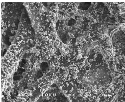
Microscopías electrónicas de barrido mostrando las partículas blancas de MgO entre las fibras del papel tras el tratamiento.
